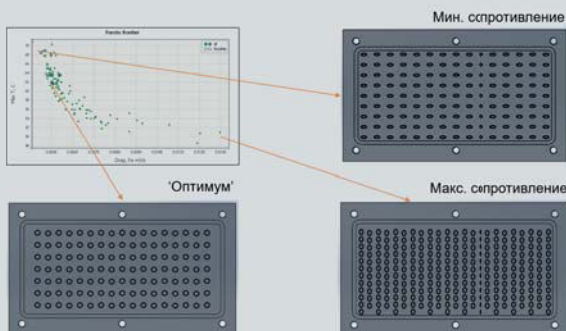
Оптимизация охлаждающей пластины транзистора при помощи FloEFD и pSeven
